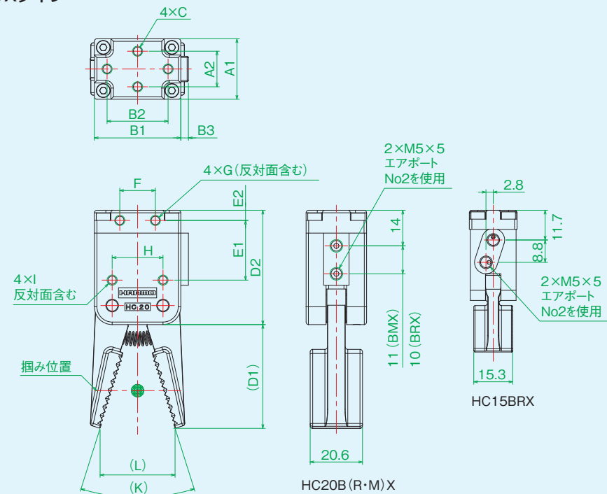
HC15X・HC20Xシリーズ外観寸法図
